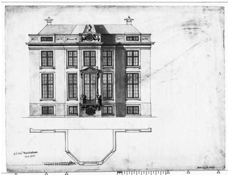
Afb. 6. Ontwerp voor een buitenhuis, niet gedateerd, gesigeneerd: H:d:Vries. 10
