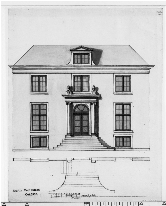
Afb. 3. Ontwerp voor een buitenhuis, niet gedateerd, gesigineerd H:d:Vries, naast de schaalstok de aantekening voor t plijn. 7
