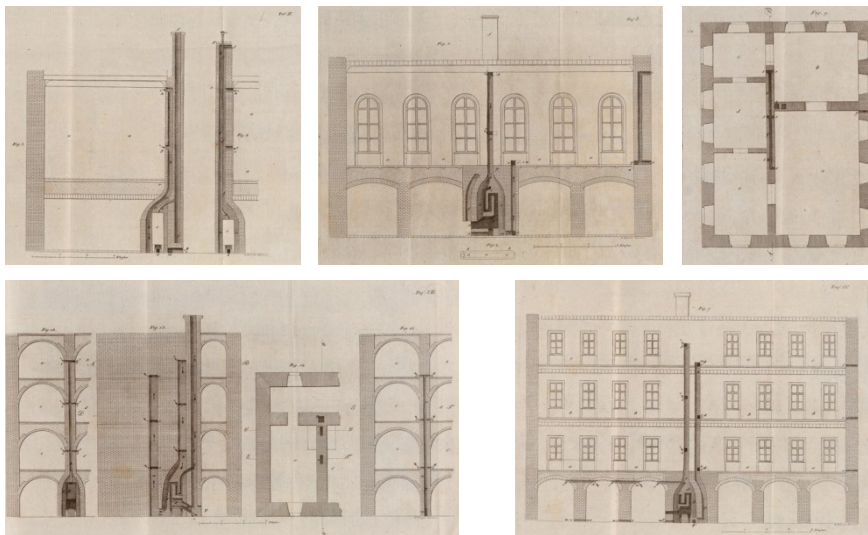
Afb. 8 t/m 12. Uitsnedes uit platen uit Die Heizung mit erwärmter Luft (1823), Paul Traugott Meißner.
