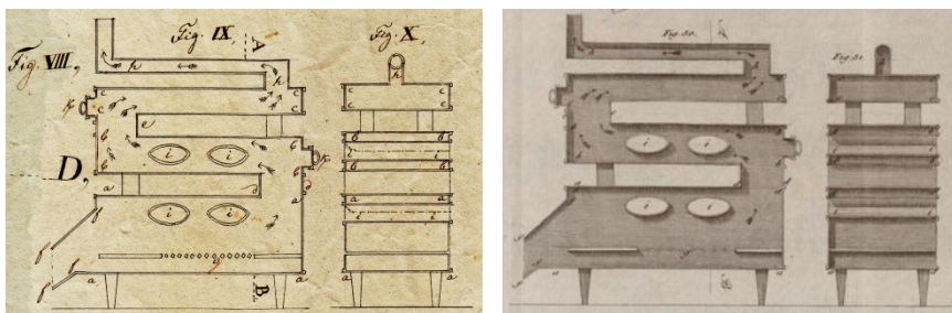
Afb. 13. Doorsneden van de oven als op het ontwerp van Übbing uit 1825 en afb. 14. Doorsneden van de oven als in het boek van Meißner uit 1823 (rechts).
