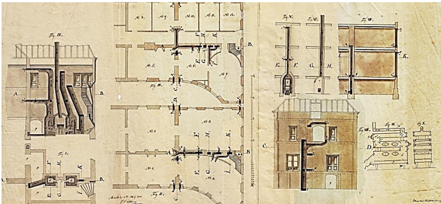
Afb. 4. Ontwerp voor warme luchtverwarming (3 mei 1825), J.T. Übbing.
